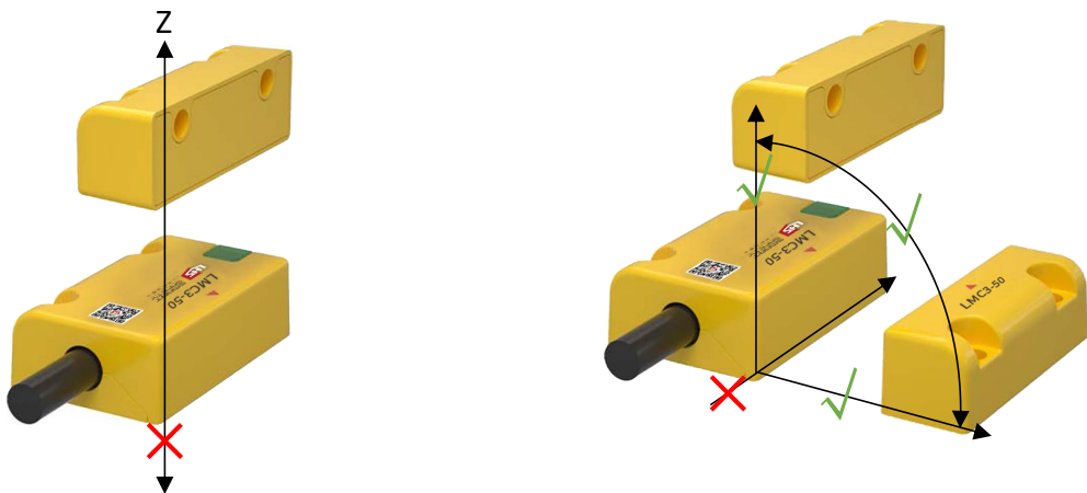
LMC3-50开关感应距离
