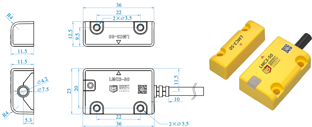
LMC3-50开关接近方向图
